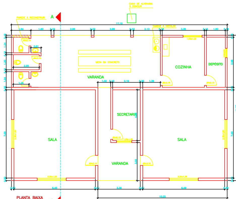
PLANTA BAIXA ESC. 1/50 AREA= 197,16m2
